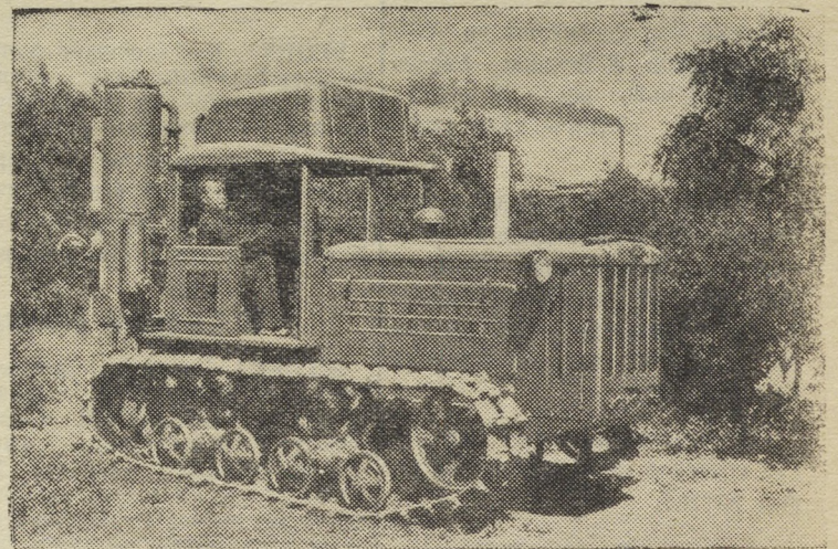
Сталинградский тракторный завод начал серийное производство гусеничного газогенераторного трактора ГБ-58, работающего на древесных чурках и брикетах торфа.
