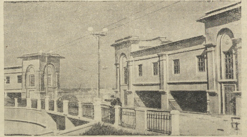
Ставропольский край. На строительстве Кубань-Егорлыкской оростительной системы. На снимке: головной шлюз Право-Егорлыкского канала. Фото Г. Аракельяна. Прессклише ТАСС.
