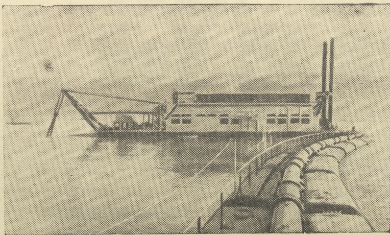
В район строительства Куйбышевской гидроэлектростанции прибыл из Сталинграда самый крупный в мире земснаряд „Сталинградский-1“, производительностью 1000 кубометров грунта в час.
