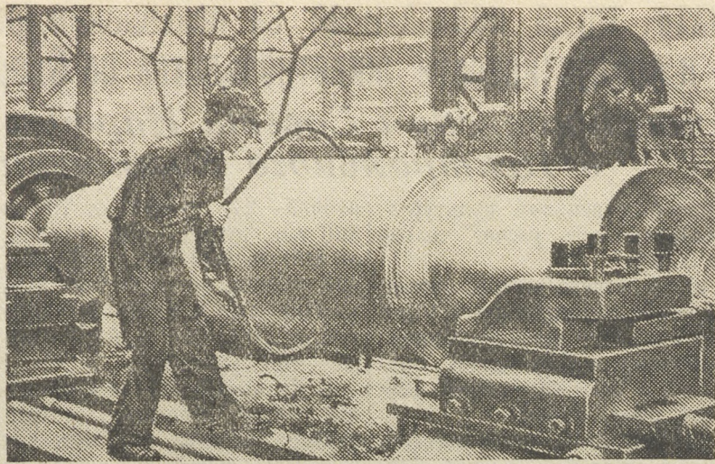
Обточка вала блюминга в механическом цехе Уралмашзавода. Слева токарь А. П. Коновалов.
