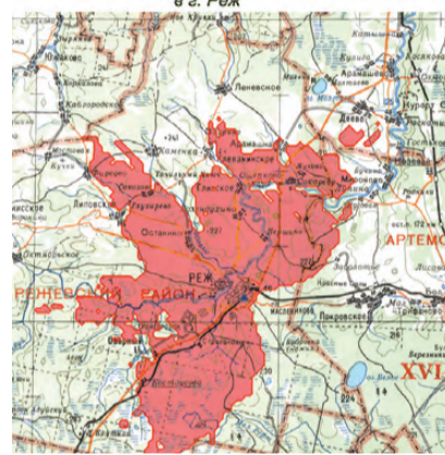
Расчетная зона обслуживания цифрового передатчика 46 ТВК пакет РТРС 1 в г. Реж
