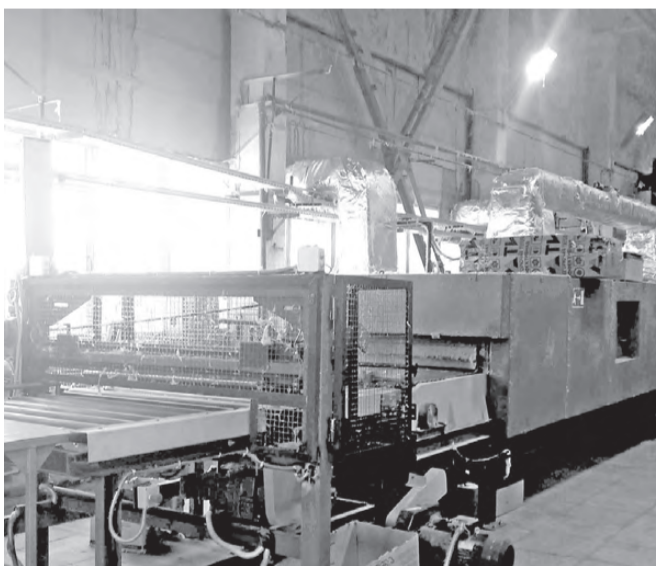
Новая линия позволила на 40% увеличить выпуск плит и картона из базальтового волокна.
