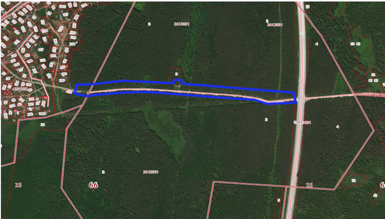
Рис. 2. Схема размещения территории планируемого размещения линейного объекта на кадастровом плане территории
