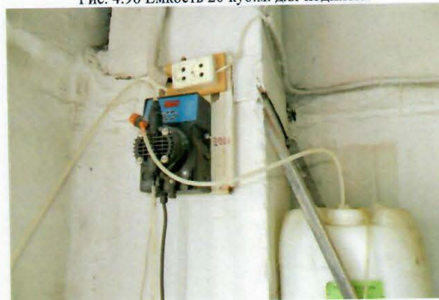
Рис. 4.98 Дозатор хим.водоподготовки с канистрой реагентов СК-110
