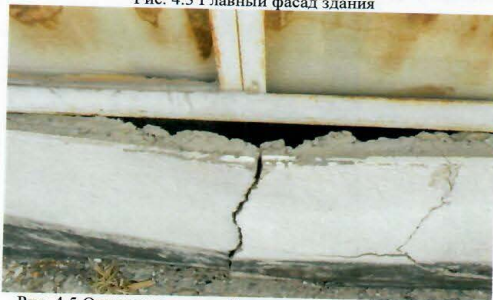
Рис. 4.5 Отслоение внешней части стены оконного проема
