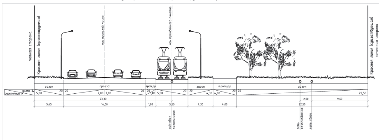
Поперечный профиль пр. Ленинградский с утвержденными и проектируемыми красными линиями. М 1:200
