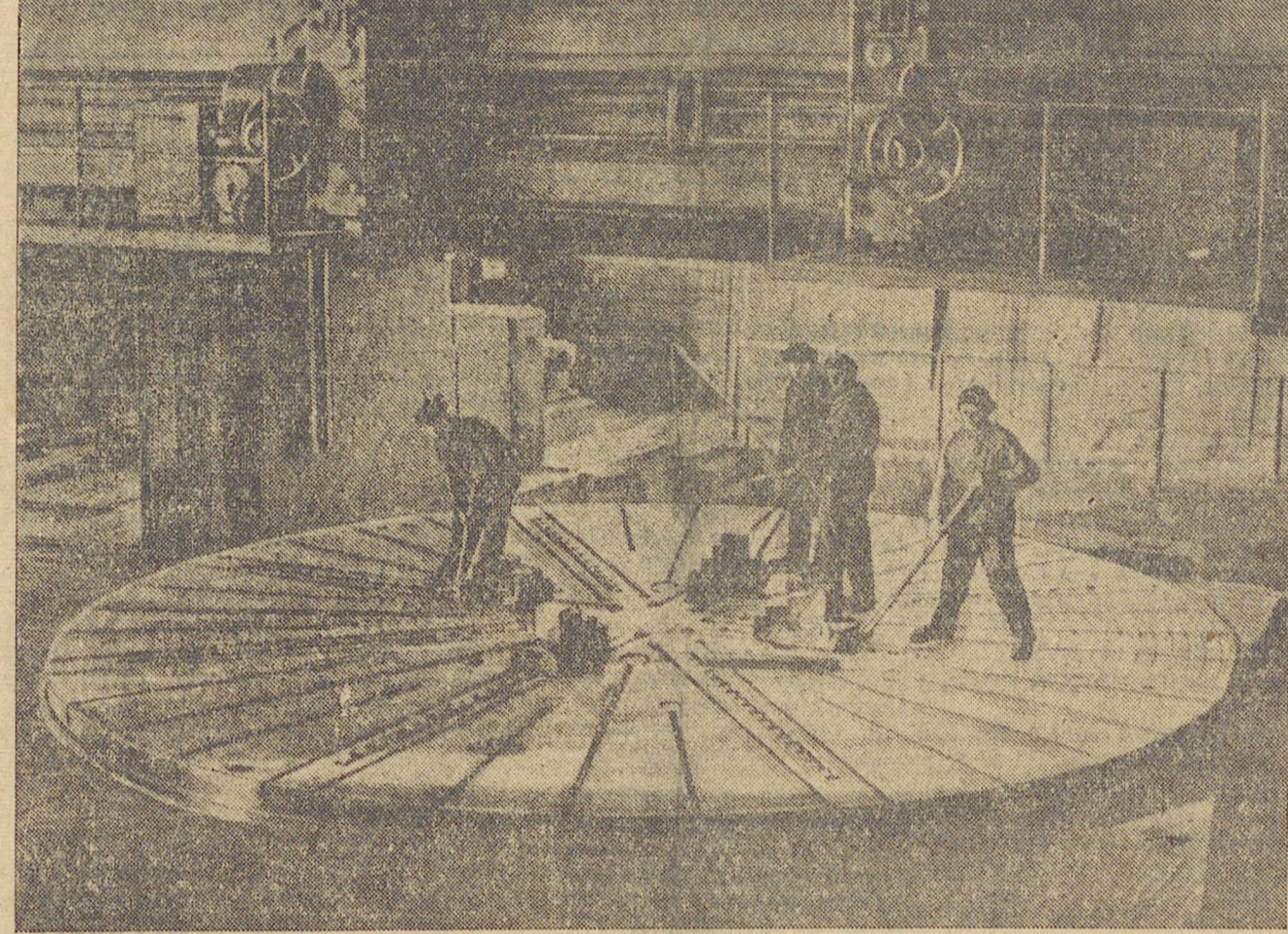
Уральский завод тяжелого химического машиностроения. На снимке: монтаж карусельного станка с 8-метровой планшайбой для обточки больших деталей. Фото Т. Стафеевой.
