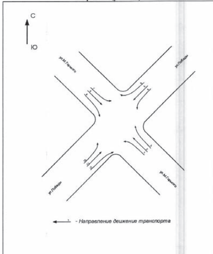
Схема направлений движения на перекрестке улиц Победы – Максима Горького (узел Б2)
