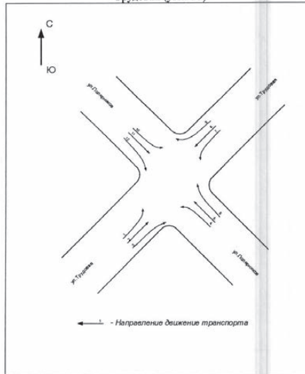
Схема направлений движения на перекрестке улиц Полярников - Трудовая (узел Б5)
