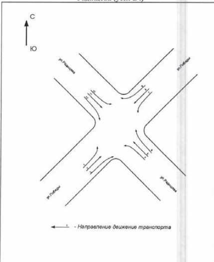
Схема направлений движения на перекрестке улиц Победы - Радищева (узел Б4)
