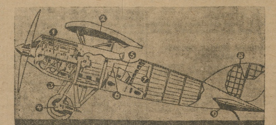
Продольный разрез истребителя «Ньюпорт де-Лаж» — самого мощного французского самолета. 1. Мотор в 500 лошадиных сил, 2. Крылья, 3. Охладитель, 4. Скрытая ось для посадочных колес, 5. Место для летчика, 6. Руль, 7. Конструкция остова, 8. Задний регулятор, 9. Регулятор высоты.
