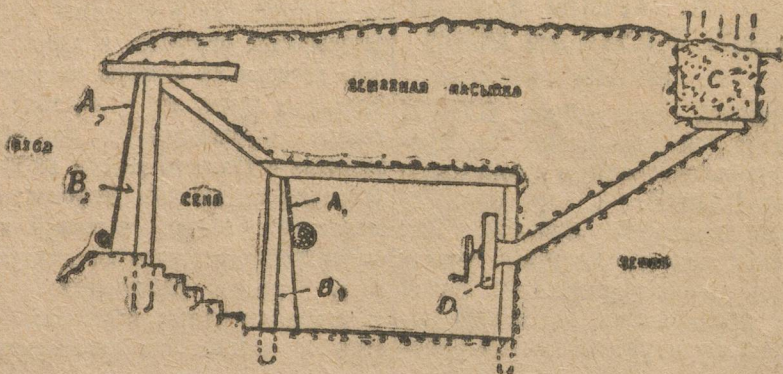
Устройство газобезопасной А 1 и А 2 —внутренняя наружная занавеси; В 1 и В 2 —рамы; С—фильтр для очистки воздуха; Д—приспособление для продувания воздуха через помещение газобезопасной (вентилятор).
