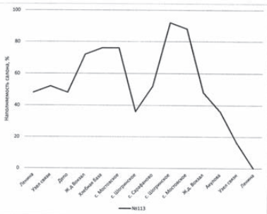
Рисунок 2 – График наполненности маршрута в зависимости от максимальной вместимости транспортного средства
