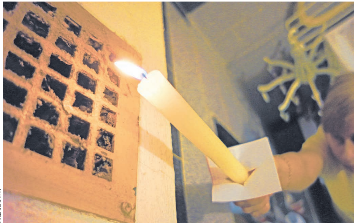
Горящая свеча поможет определить, работает вентиляция или нет.
