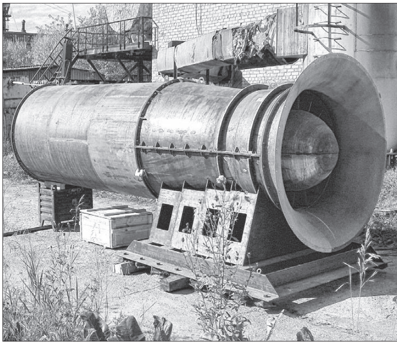
Устройства защиты систем вентиляции были изготовлены на комбинате «Электрохимприбор» соседнего города Лесного / ФОТО ОАО «ВЕНТА»
