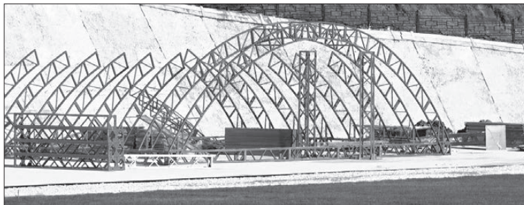
Строительство стадиона в п. Пионерском.
