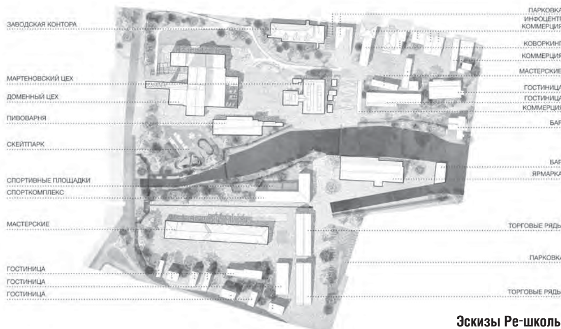
ГЕНЕРАЛЬНЫЙ ПЛАН
