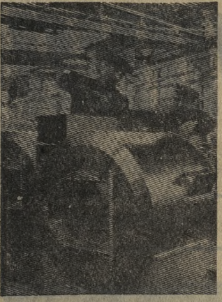
Развивается и совершенствуется служба быта в нашей стране. Московский машиностроительный завод «Коммунальник» выпускает различные машины и оборудование для механизированных прачечных. Предприятие также экспортирует свою продукцию в Японию, Болгарию, Францию, ФРГ, Турцию, Египет и другие страны мира. На снимке: в цехе сборки автоматизированных стиральных машин. Фото В. Кошевого.
