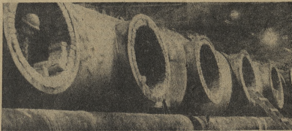
РЕКОНСТРУКЦИЯ И КАПИТАЛЬНЫЙ РЕМОНТ СТАНА «30-102»
