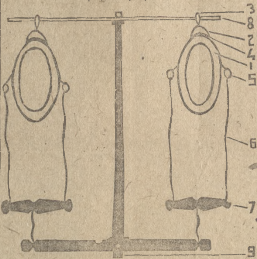
1. Шора из пожарного рукава или холста шириной 1—1½ вер. 2. Деревянная кобылка. 3. Кольцо на кобылке. 4. Кошма подложенная под кобылку. 5. Кольцо у шоры. 6. Постромка. 7. Валок. 8. Деревянная перекиладина. 9. Прицепляется плуг.
