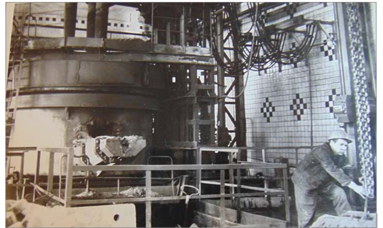
Литейный участок МЛЦ. Сталеплавильная печь.
