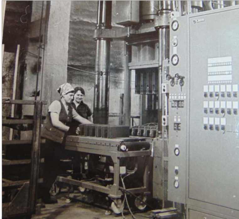
Ручной съём полуфабриката с пресса «Лайс» в цехе №2.
