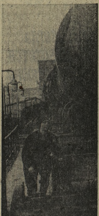
ВОЛЬСК. (Саратовская область). На крупнейшем заводе «Большевик» пущена новая, одиннадцатая по счету технологическая линия производства цемента. Вращающаяся печь этой линии — 185 метров длины. Она способна выдать 72 тонны клинкера в час. НА СНИМКЕ: смазчик мотористка комсомолка Лида Спиридонова. Она следит за работой новой 185-метровой печи. Фото Е. СОКОЛОВА. Фотохроника ТАСС.
