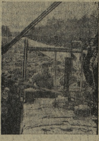
КОМИ АССР. На строительстве газопровода «Сияние Севера» идет опробование готового участка Вуктыль-Ухта протяженностью почти в 200 километров. На других отрезках трассы также уложены в траншеи десятки километров труб. НА СНИМКЕ: за работой один из лучших мастеров трубоуладчиков Иван Хайбин. Фото С. ГУБСКОГО. Фотохроника ТАСС.
