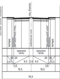
МАГИСТРАЛЬ ОБЩЕОБЛАСТНОГО ЗНАЧЕНИЯ РЕГУЛИРУЕМОГО ДВИЖЕНИЯ (проектируемый путепровод)
