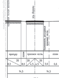
УЛ. ПАРКОВЕНКО от ул. Железнодорожной до ул. Победы (проектируемый профиль)
