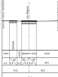
УЛ. ПАРКОВЕНКО от ул. Тилова до ул. Железнодорожной (проектируемый профиль)
