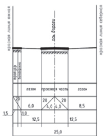
МАГИСТРАЛЬ ОБЩЕОБЛАСТНОГО ЗНАЧЕНИЯ РЕГУЛИРУЕМОГО ДВИЖЕНИЯ (ул. Тилова)
