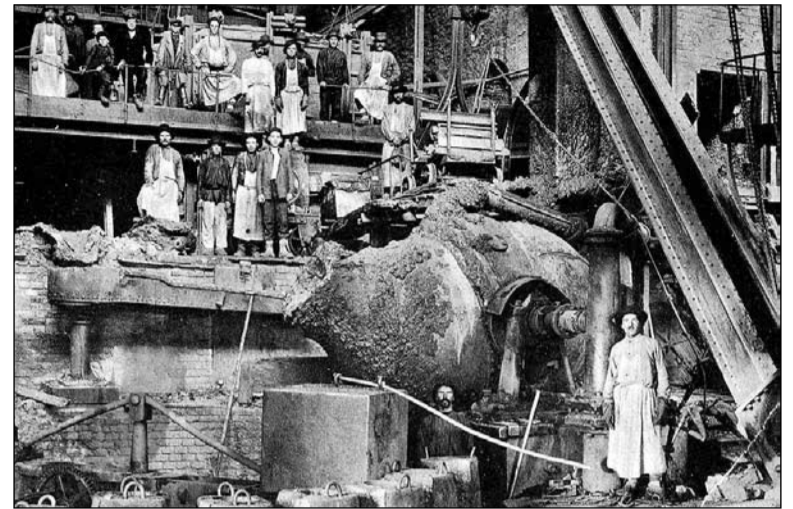
Внутренний вид бессемера.
