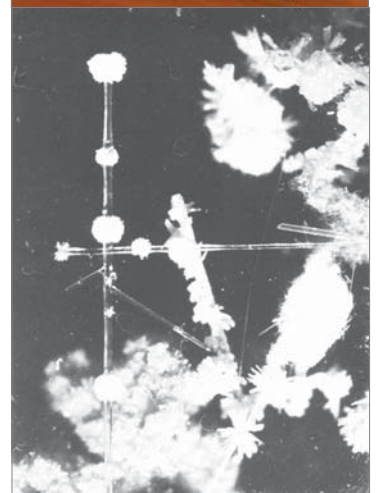
«Снежки» из форстерита и игольчатый периклазовый «иней».
