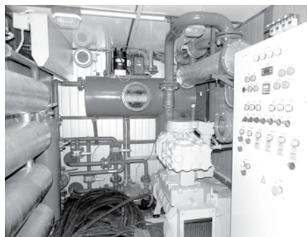
Так выглядит внутреннее оборудование машины для восстановления трансформаторного масла.
