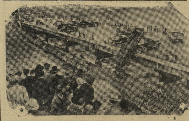
19 июня строители Братской ГЭС закончили перекрытие Ангары. Фото В. Савостянова.
