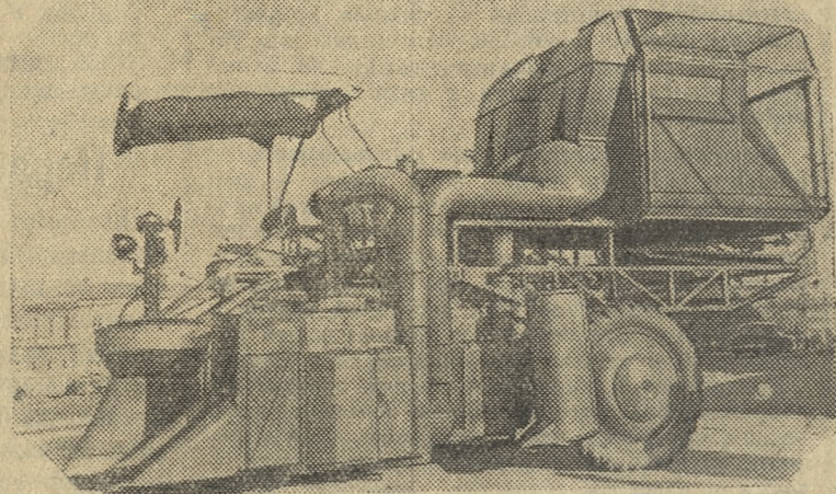
Узбекская ССР. Завод «Ташсельмаш» приступает к выпуску горизонтально-шпиндельных и вертикально-шпиндельных хлопкоуборочных машин. В 1959 году должно быть изготовлено 1350 таких машин.
