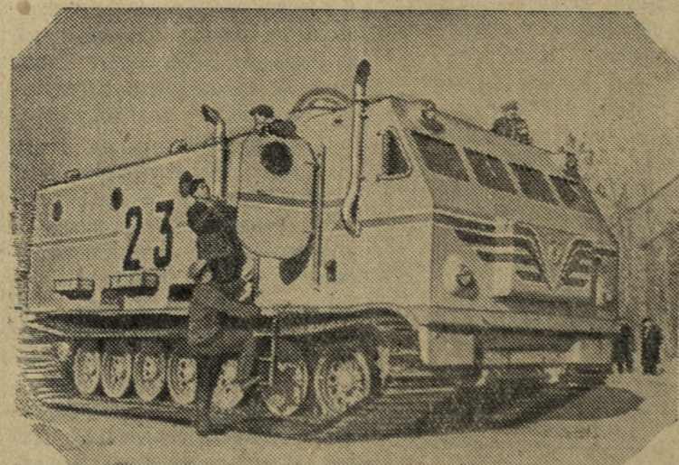
Харьков. Новые трудовые подарки в честь XXI съезда КПСС готовят коллективы предприятий города. Для четвертой Антарктической экспедиции машиностроители подготовили три мощных тягача большой проходимости. На снимке: общий вид антарктического тягача.
