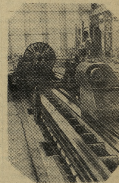
КНР. На Харбинском заводе силового оборудования закончено строительство цеха турбогенераторов. Здесь будут производиться электрические машины мощностью 200 — 300 тысяч киловатт.
