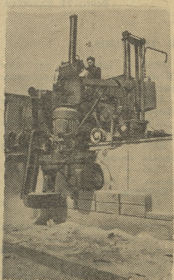
Москва. Коллектив завода «Строммашина» создал новую камнерезную машину «СМ-543» для добычи штучного камня в карьерах малой мощности высокоуступчатым методом.
