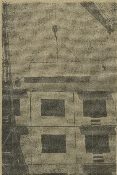
Заканчивается монтаж четвертого этажа второго по счету дома, сделанного из новейшего строительного материала пенобетона. Эти дома первые в Советском Союзе.
