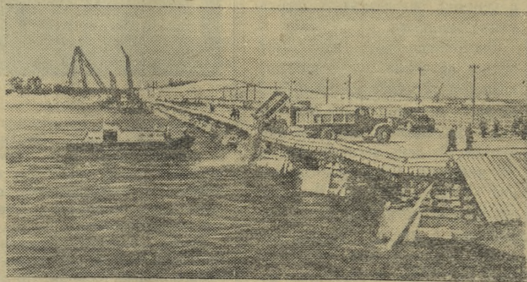
ГОРЬКОВСКАЯ ОБЛАСТЬ. Для перекрытия русла Волги на строительстве Горьковской гидроэлектростанции сооружен понтонный мост шириной в 20 метров и длиной в 300 метров, с которого автосамосвалы сбрасывают камень. НА СНИМКЕ: общий вид понтонного моста.
