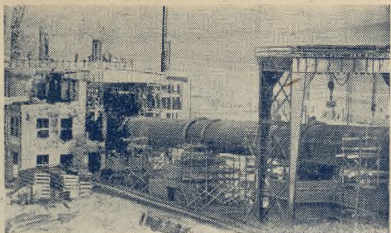
Крымская область. Недалеко от города Бахчисарая сооружается межколхозный цементный завод. Строители взяли обязательство сдать первую очередь предприятия в эксплуатацию в конце декабря. К этому времени первая вращающаяся печь длиной 101 метр и диаметром 3 метра даст первый цемент. Началось также строительство второй очереди завода. НА СНИМКЕ: общий вид строительства Крымского межколхозного цементного завода.
