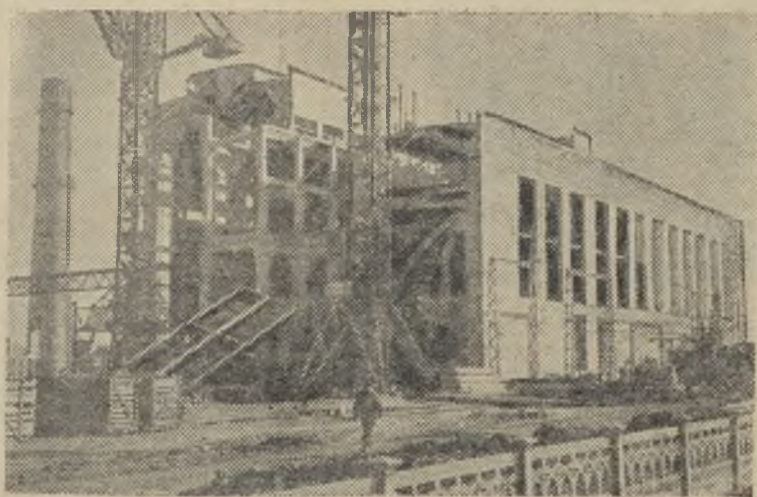
В близ Симферополя ведется опытно-показательное строительство ГРЭС. Сооружения электростанции возводятся из сборного железобетона и крупных блоков. В этом году будет завершено строительство первой очереди.
