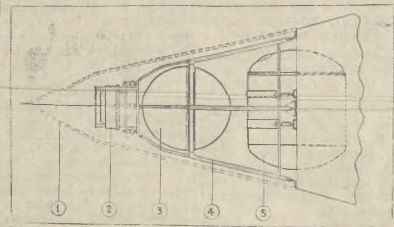
Схема размещения аппаратуры второго искусственного спутника: 1. Защитный конус, сбрасываемый после выведения спутника на орбиту. 2. Прибор для исследования ультрафиолетового и рентгеновского излучения Солнца. 3. Сферический контейнер с аппаратурой и радиопередатчиками. 4. Силовая рама для крепления аппаратуры. 5. Герметическая кабина с подопытным животным.
