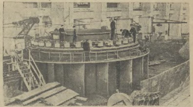
Украинская ССР. Коллектив Харьковского турбинного завода имени Кирова изготовил 8-ю, последнюю, гидротурбину мощностью 90 тысяч киловатт для Иркутской ГЭС. На снимке: подготовка к демонтажу перед отпавкой в адрес Иркутской ГЭС направляющего аппарата 8-й гидротурбины. Фото Е. Андреева. Фотохроника ТАСС.
