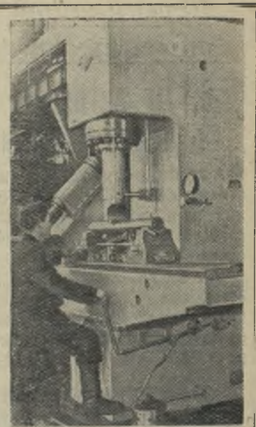
Чкаловский завод гидравлических штамповочных пресов увеличивает выпуск продукции, осваивает производство пресов новых конструкций. В декабре 1956 года здесь был изготовлен новый пресс П-417 с усилием давления в 100 тонн для правки заготовок. На снимке: слесарь А. И. Шенн проверяет пресс П-417 для правки заготовок. Фото Б. Клиппингера. Фотохроника ТАСС
