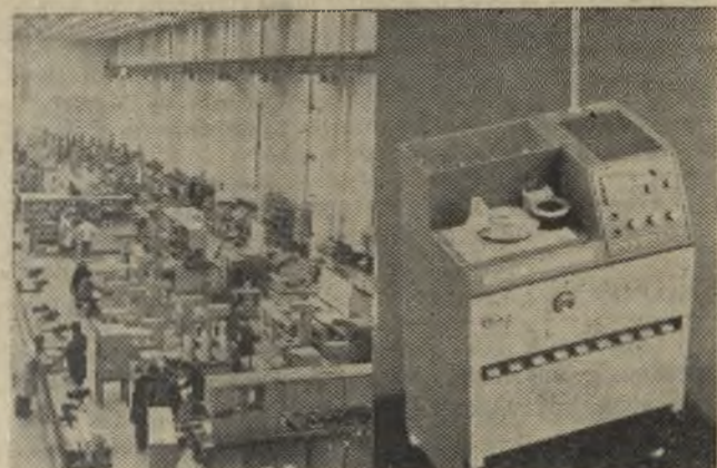
Недавно на московском инструментальном заводе «Калибр» освоили выпуск опытных образцов сортирующих автоматов для шарикоподшипниковой промышленности. Новинка позволяет высвободить за смену до 50 рабочих, значительно сократить трудоемкие процессы. Годовой экономический эффект от ее применения составит пятьдесят восемь тысяч рублей.
